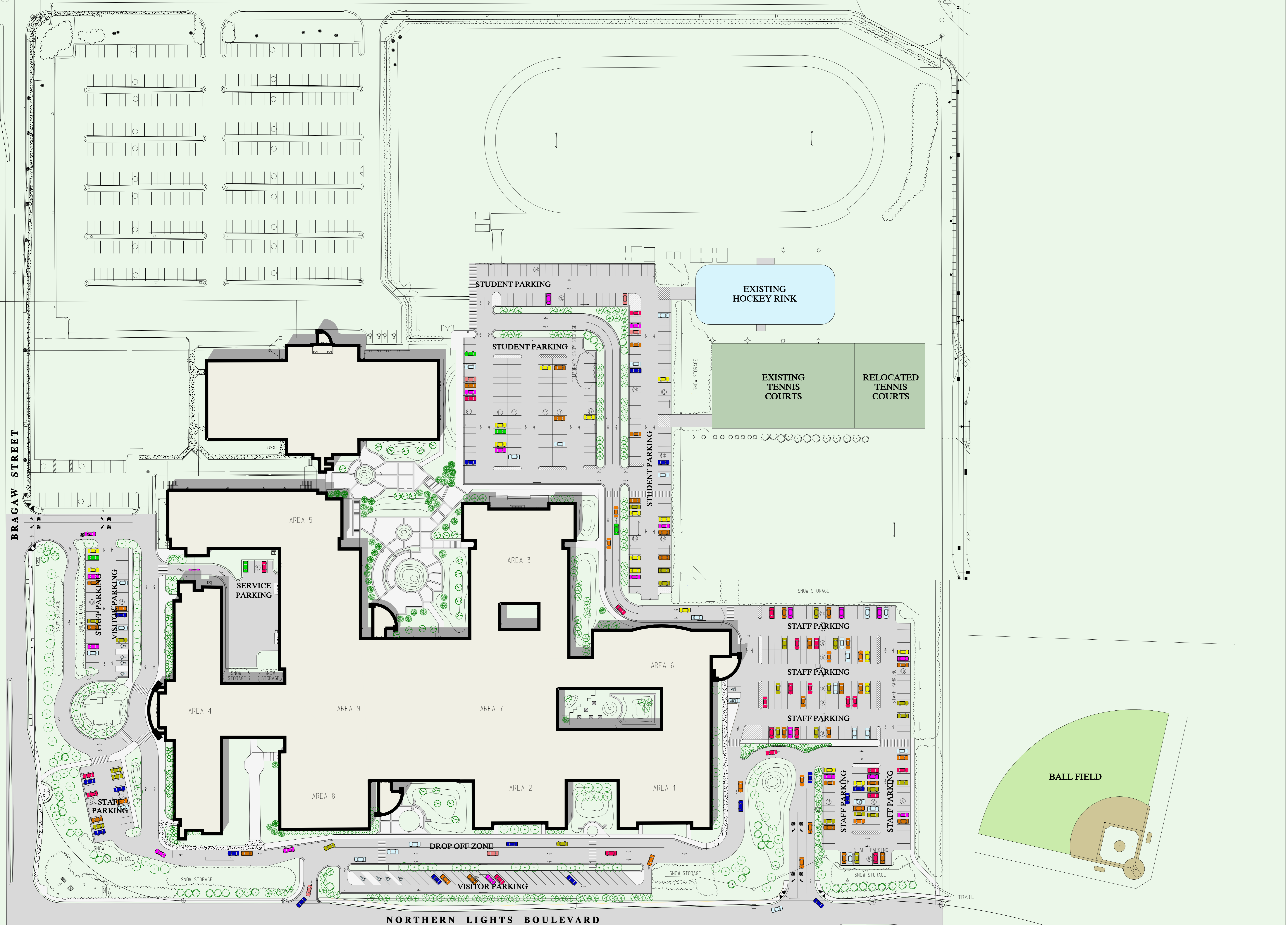
1 Phases 1, 2, & 3 Site Plan
